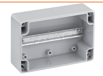
Точки кріплення DIN-рейки або монтажної пластини розміщені у прийнятних на ринку позиціях. У разі необхідності, за допомогою ультразвукового зв'язування, виробник розмістить їх у відповідності до Ваших побажань
