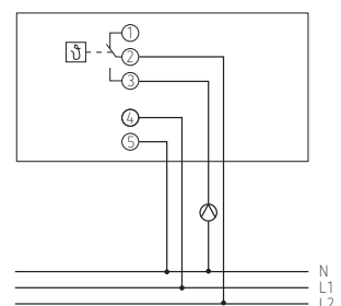
RAMSES 722, RAMSES 782, RAMSES 721, RAMSES 725
