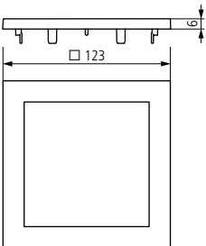
PlanoCentro UWH-A KNX
