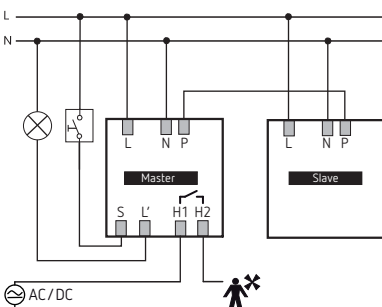
thePrema P360-101 E, thePrema P360 Slave E
