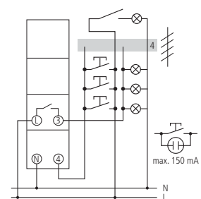
ELPA 6, ELPA 6 plus, ELPA 7
