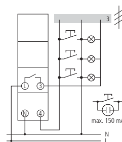
ELPA 6, ELPA 6 plus, ELPA 7
