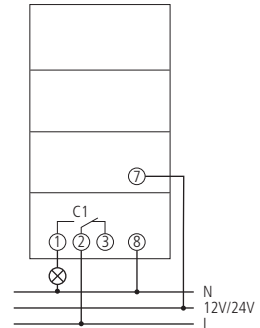
SUL 181 h 12 V, SUL 181 h 24 V
