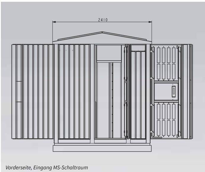
Ausführung begehbare MS- und NS-Schalraum, nicht begehbare Transformatorraum
