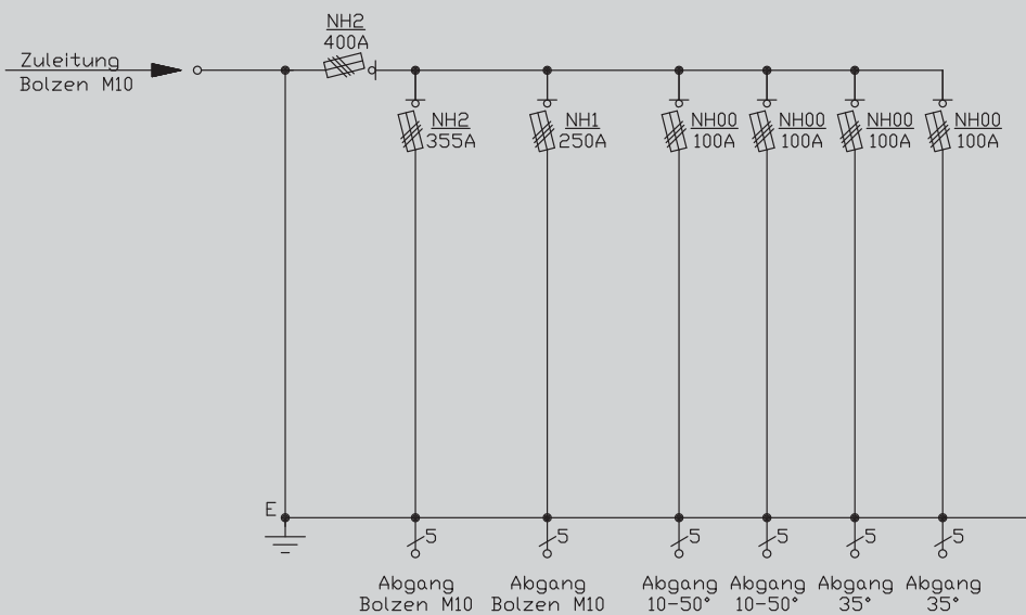
Prinzipschaltbild WGV0080
