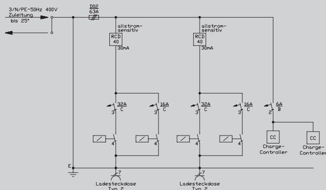
Prinzipschaltbild E21X01AP0910
