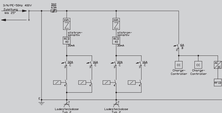
Prinzipschaltbild E51C011429B0
