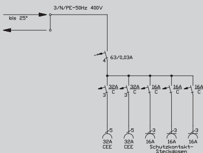
Prinzipschaltbild 6913001
