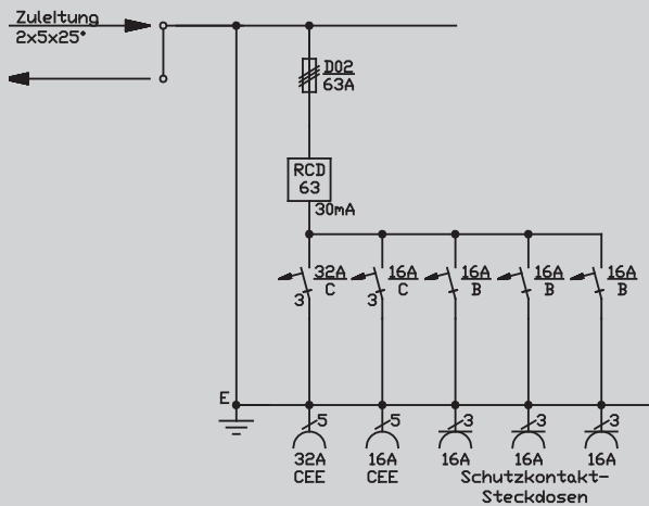
Prinzipschaltbild 83210000
