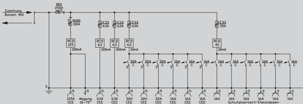
Prinzipschaltbild 83100572
