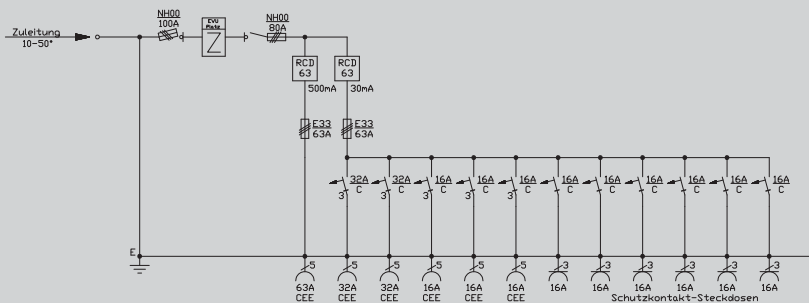
Prinzipschaltbild WAV0179
