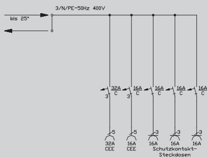
Prinzipschaltbild 6983017
