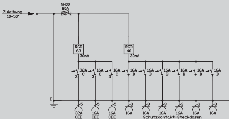
Prinzipschaltbild 83210100
