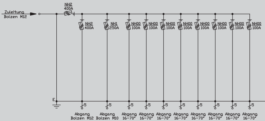
Prinzipschaltbild 83216500
