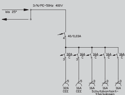
Prinzipschaltbild 6823009
