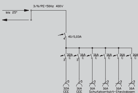
Prinzipschaltbild 6993103
