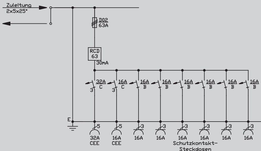
Prinzipschaltbild 83215000
