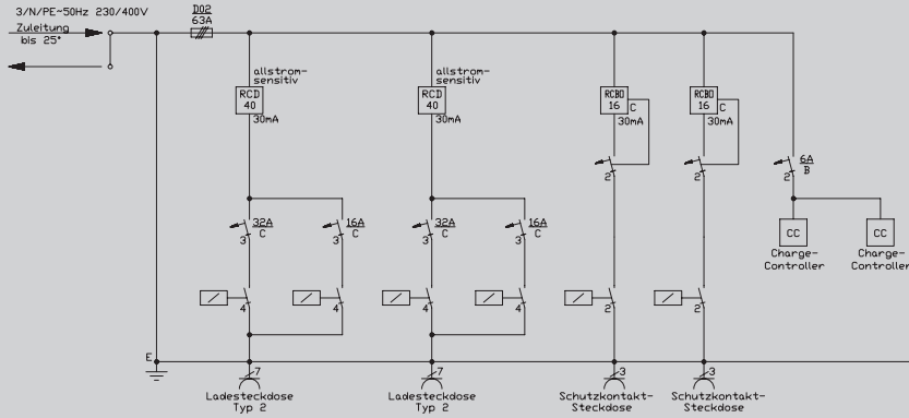
Prinzipschaltbild E48X01AE096A
