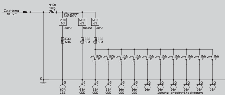
Prinzipschaltbild WV0434A
