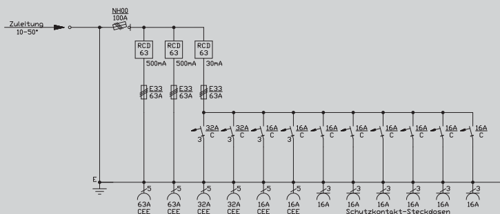
Prinzipschaltbild WV0434
