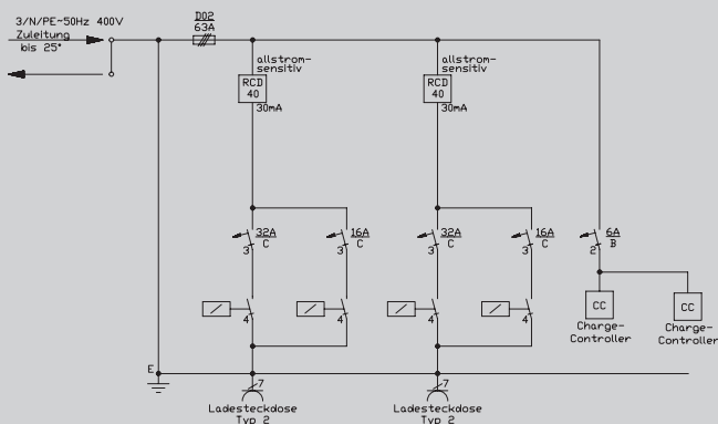
Prinzipschaltbild E41X01AE0960
