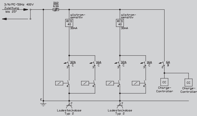
Prinzipschaltbild E41X01AP0960
