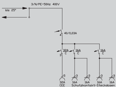
Prinzipschaltbild 6821202
