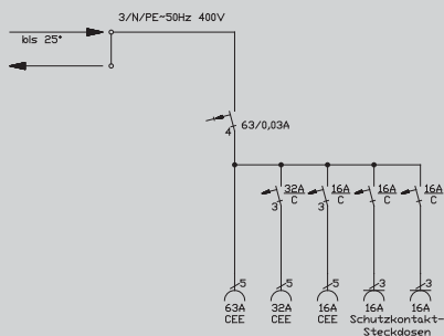
Prinzipschaltbild 6894418
