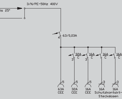
Prinzipschaltbild 6824403x7
