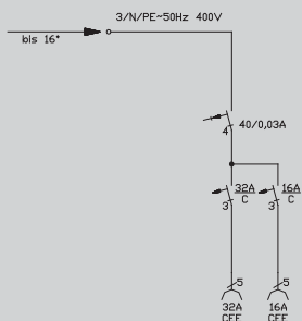
Prinzipschaltbild 6923015
