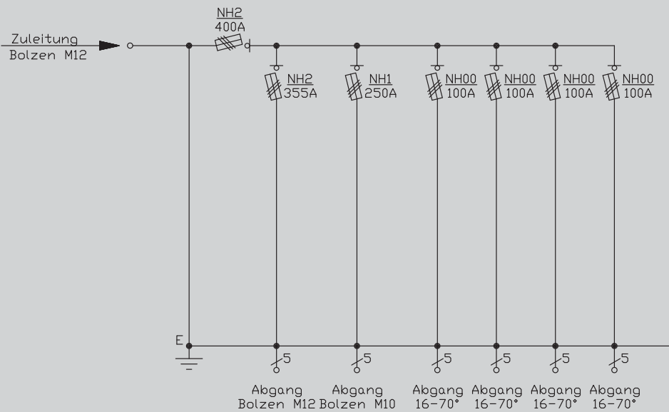
Prinzipschaltbild WGV0082
