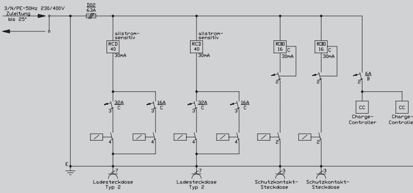
Prinzipschaltbild E28X01AE091A
