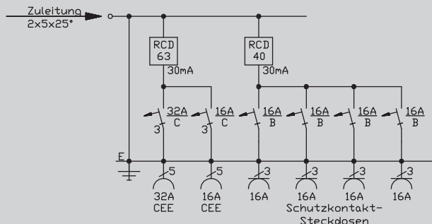
Prinzipschaltbild 8AP59580
