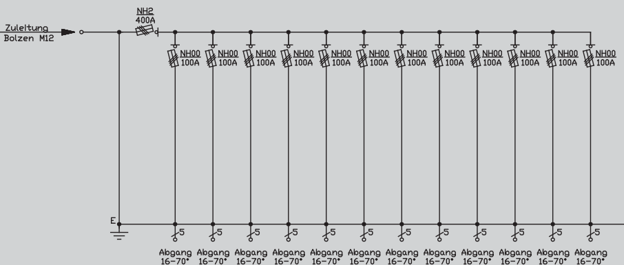
Prinzipschaltbild 83216600
