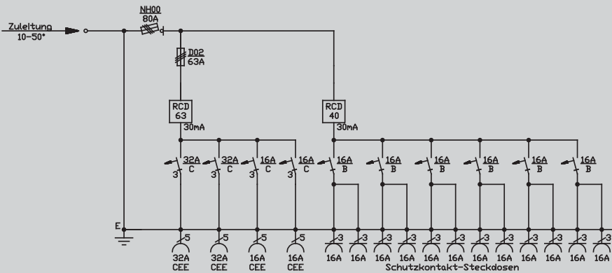
Prinzipschaltbild 83215100
