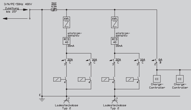
Prinzipschaltbild E41X01A249B0
