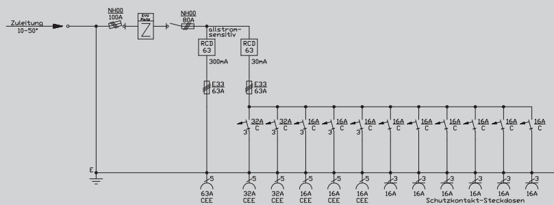
Prinzipschaltbild WAV0179A
