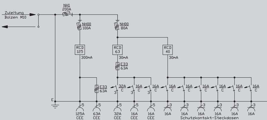
Prinzipschaltbild 83100494
