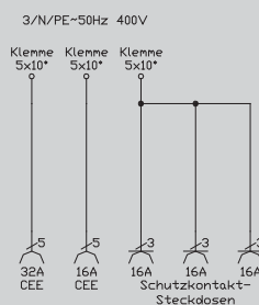
Prinzipschaltbild 6913001
