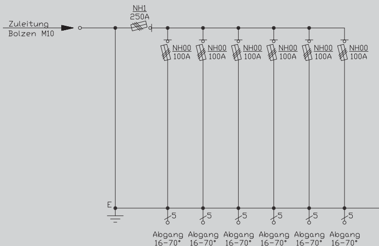
Prinzipschaltbild WGV0076
