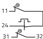
Elemento di contatto con automonitoraggio Contact block with self-monitoring
