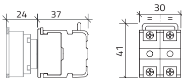
Elemento di contatto con automonitoraggio Contact block with self-monitoring
