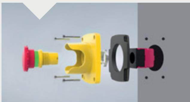
Supporto operatore per installazione ad incasso Wall-mounting support for push-button
