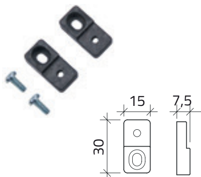
Kit di staffe di fissaggio 10 mm Set of mounting brackets 10 mm
