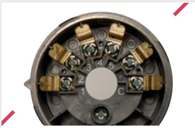
Base di alimentazione per 5 moduli luminosi con una linea comune
