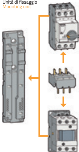
Unità di giunzione Connection unit
