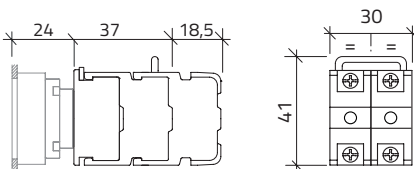
Elemento di contatto con automonitoraggio Contact block with self-monitoring
