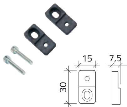
Kit di staffe di fissaggio 25 mm Set of mounting brackets 25 mm
