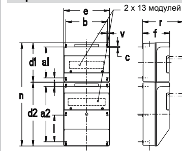
Стр. 33 689 корпус = 682 + 683 joined
