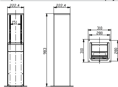
Стр. 38 Узкая стойка из нержавеющей стали
