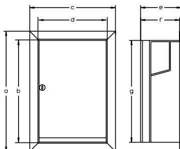
Стр. 39 Распределительный щит, утопленный монтаж
