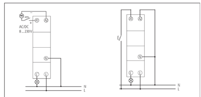
Схема подключения к сети 8...230 В AC/DC
