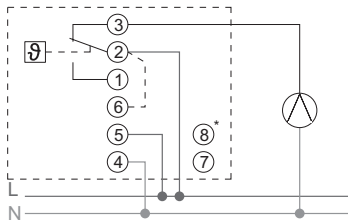
управление циркуляционными насосами и термоэлектрическими приводами клапанов
