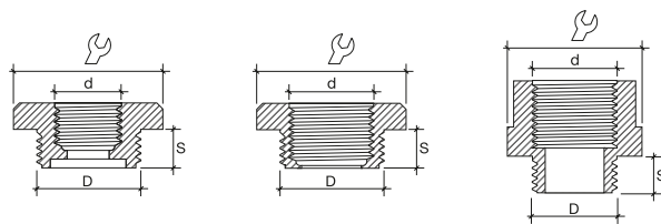
Riduzioni in plastica / plastic reducers
